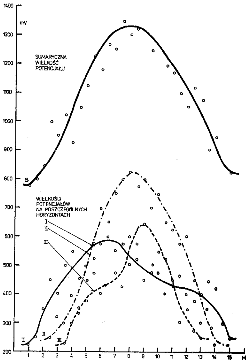
WYKRES ROZKŁADU ENERGETYCZNEGO Z TERENOWEGO POMIARU NAD CIEKAMI WIELKOŚCI POTENCJAŁÓW SPONTANICZNYCH
