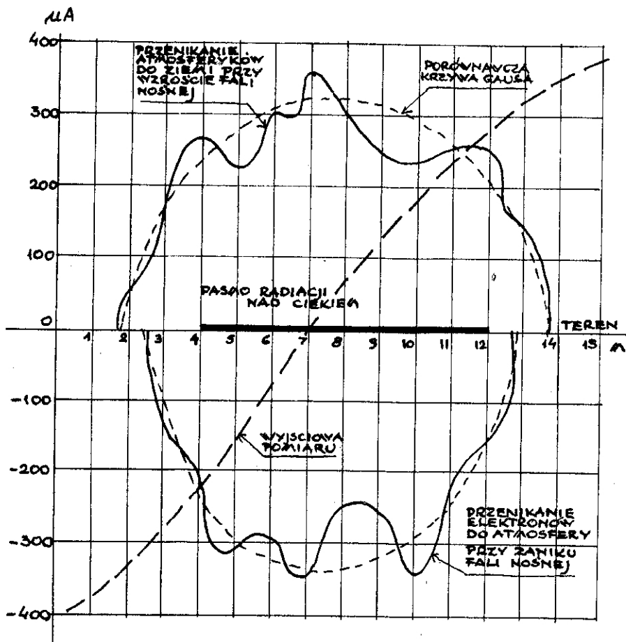
WYKRES POMIARU W POPRZEK PASMA RADIACJI PODWYŻSZONEJ WYBRANEGO PRZYKŁADOWO MIEJSCA DLA WYKAZANIA PRZEBIEGU WYKRESU W STOSUNKU DO CHARAKTERYSTYCZNEJ KRZYWEJ GAUSA
